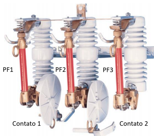
Figura 1 – Chave fusível religadora fechada.
